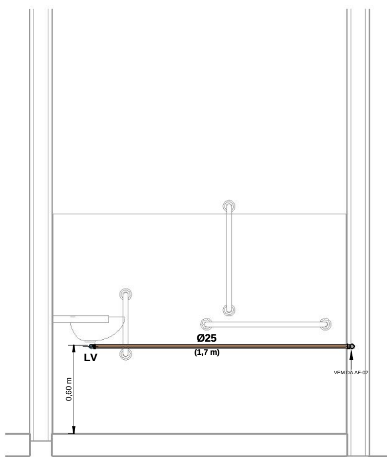
4 CORTE AF-02(LV) 1 : 25
