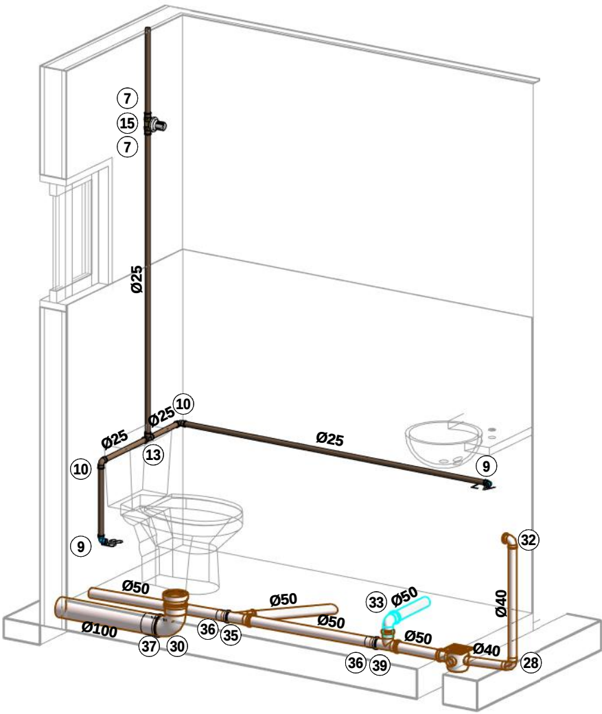
3 ISOMÉTRICA WC PNE MASC. 1 : 25
