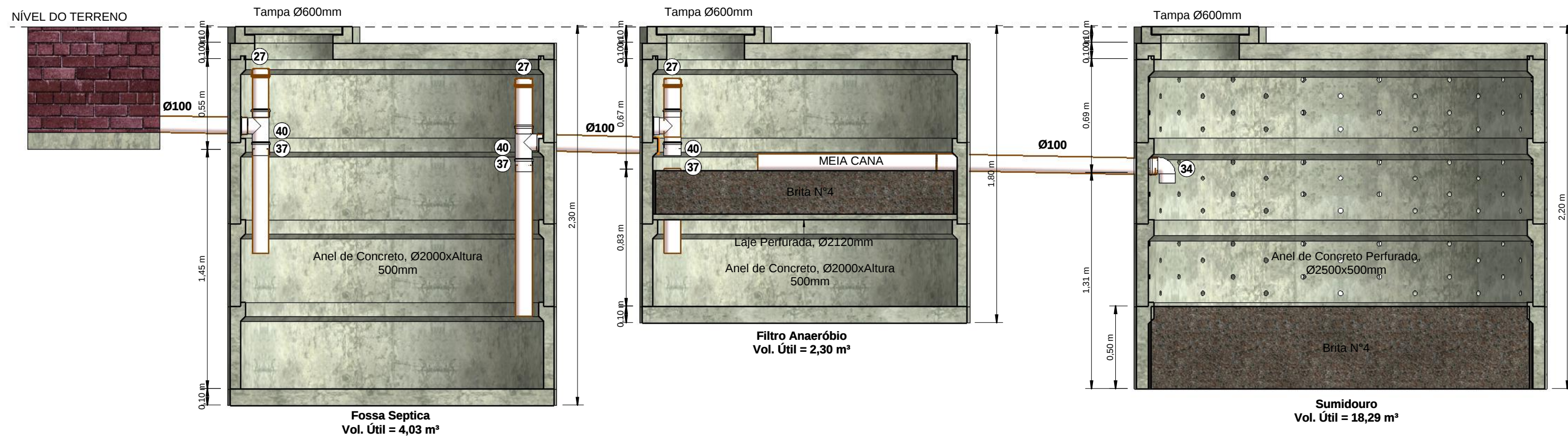
2 DETALHE SISTEMA DE TRATAMENTO DE EFLUENTE 1 : 25
