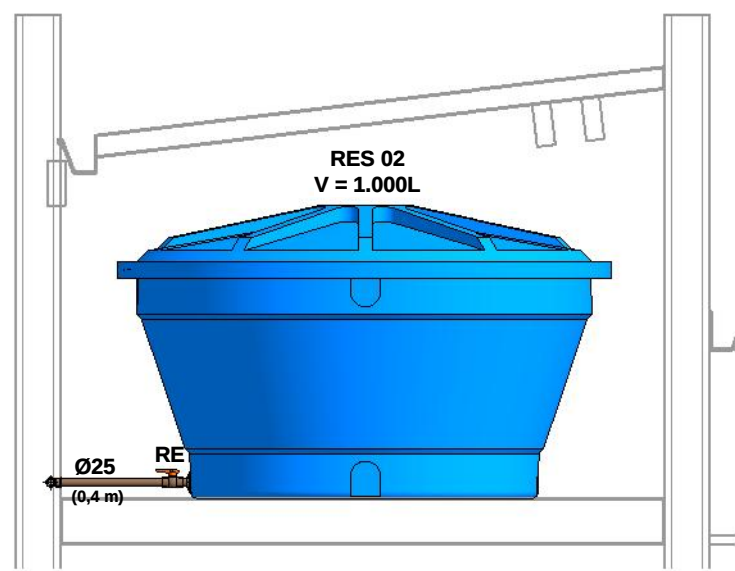
8 CORTE 8-8 1 : 25
