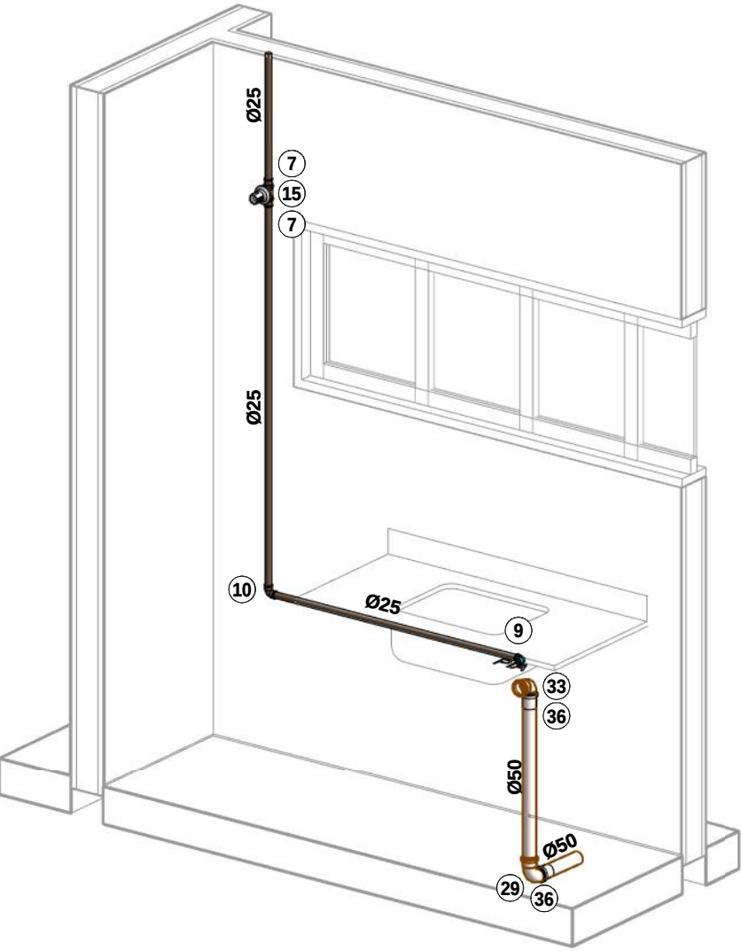
1 ISOMÉTRICA COPA/COZINHA 1 : 25
