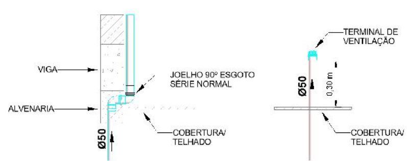
4 DET. TERMINAL DE VENTILAÇÃO 1 : 25
