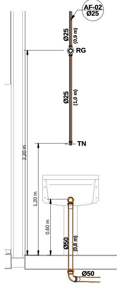
5 CORTE AF-03 1 : 25
