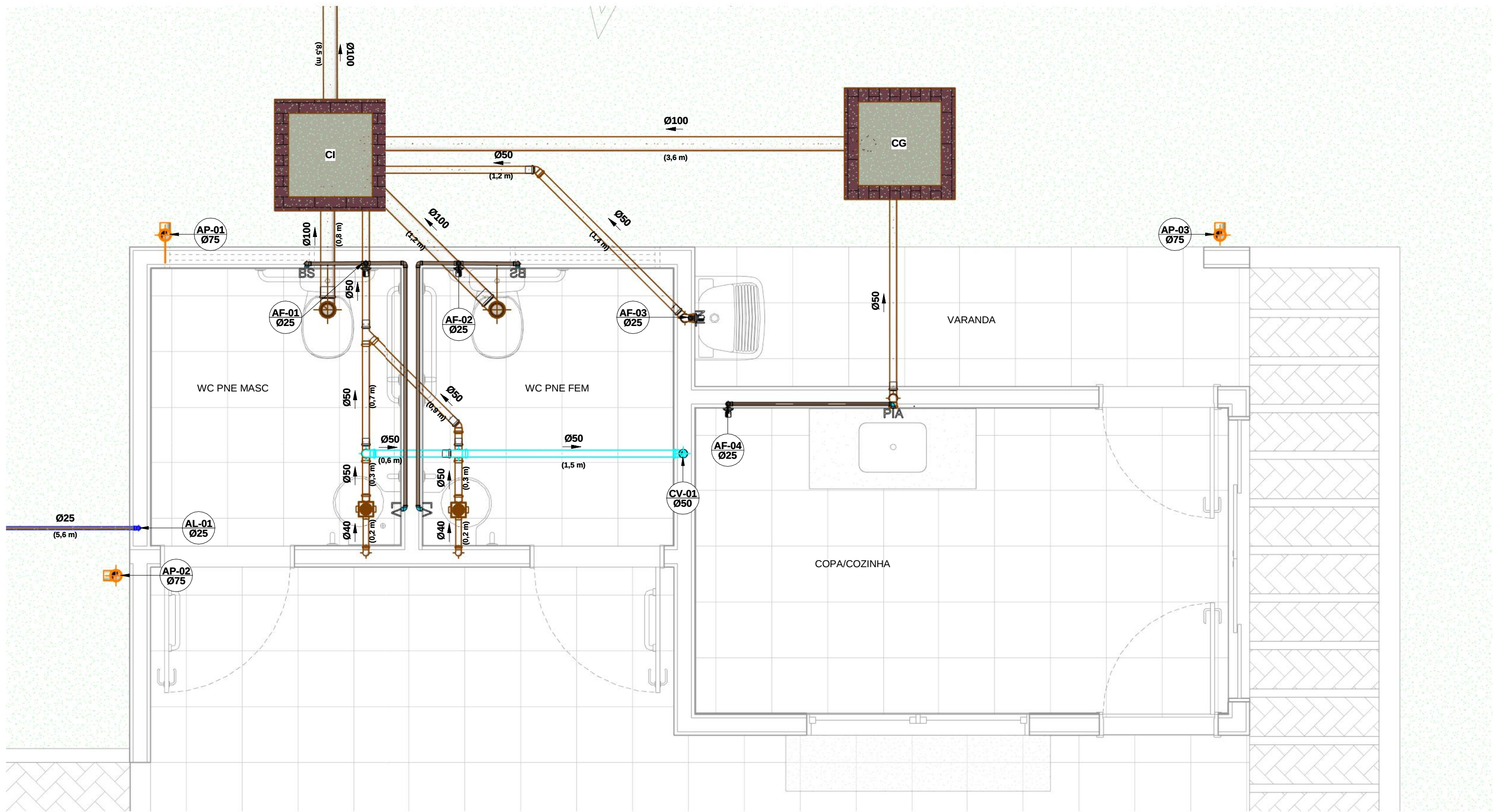
2 DET. 2 1 : 25
