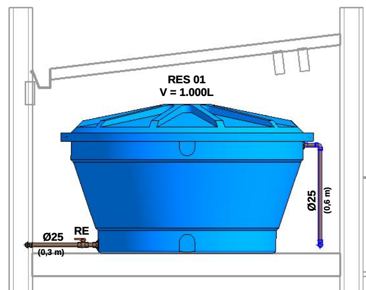
9 CORTE 9-9 1 : 25
