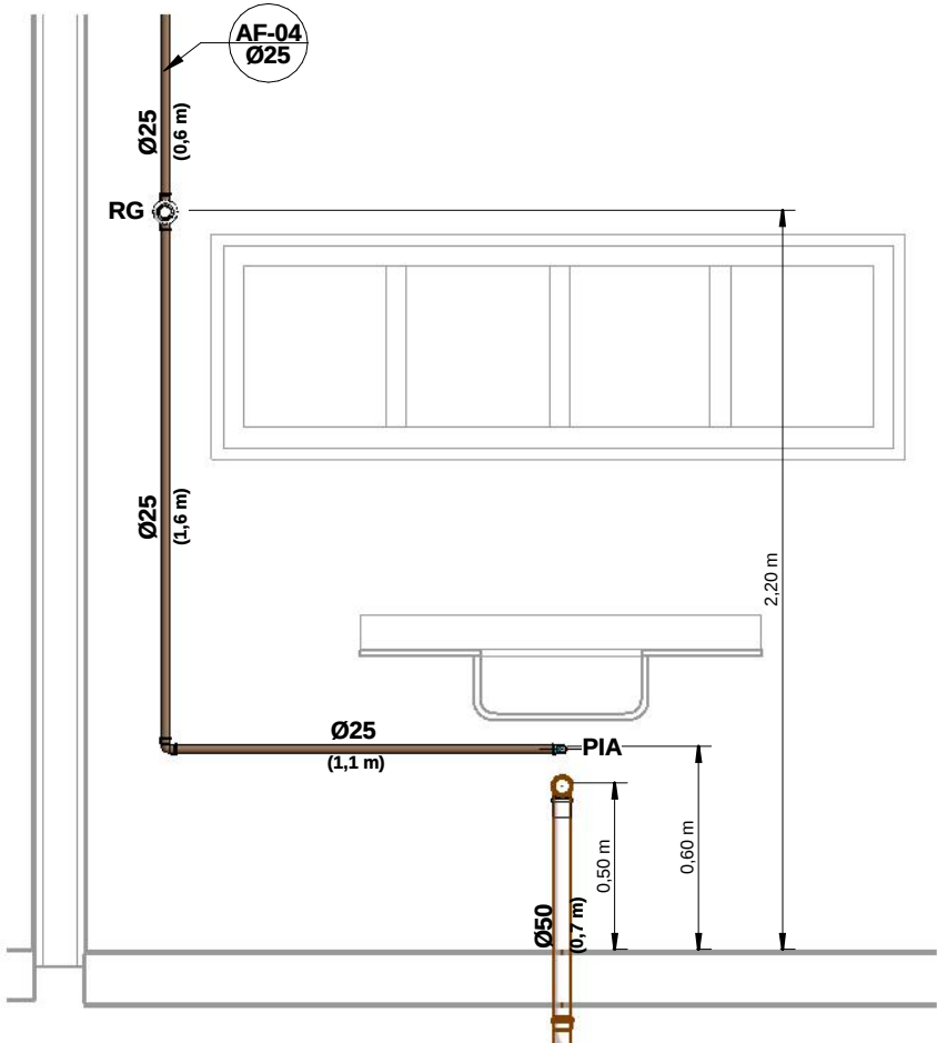
6 CORTE AF-04 1 : 25
