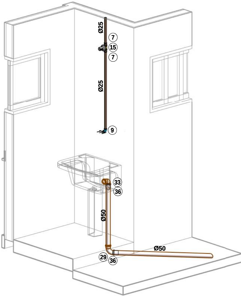
4 ISOMÉTRICA VARANDA 1 : 25
