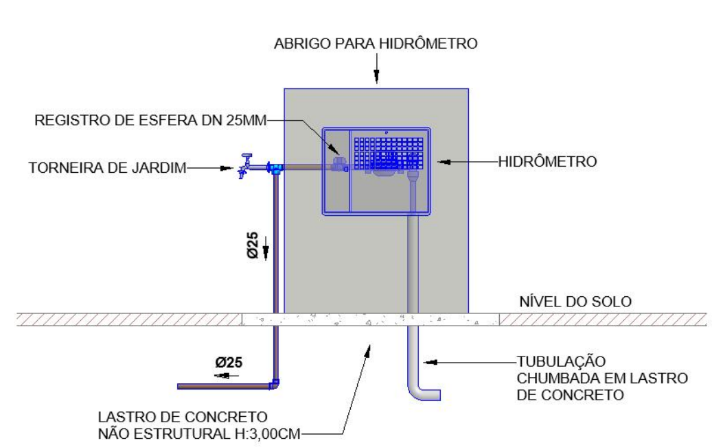
7 DET. HIDRÔMETRO 1 : 25
