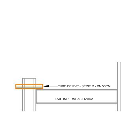
3 DET. BUZINOTE 1 : 25
