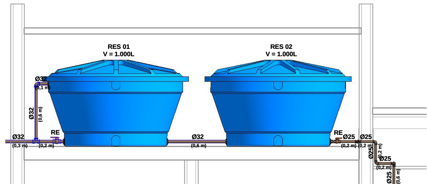
7 CORTE 7-7 1 : 25
