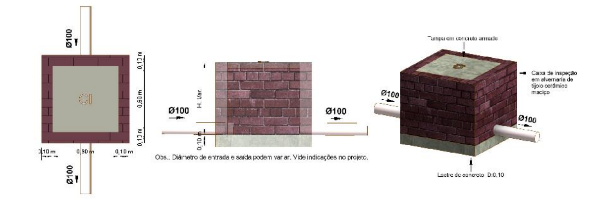
6 DET. CAIXA DE INSPEÇÃO 60X60cm 1 : 25
