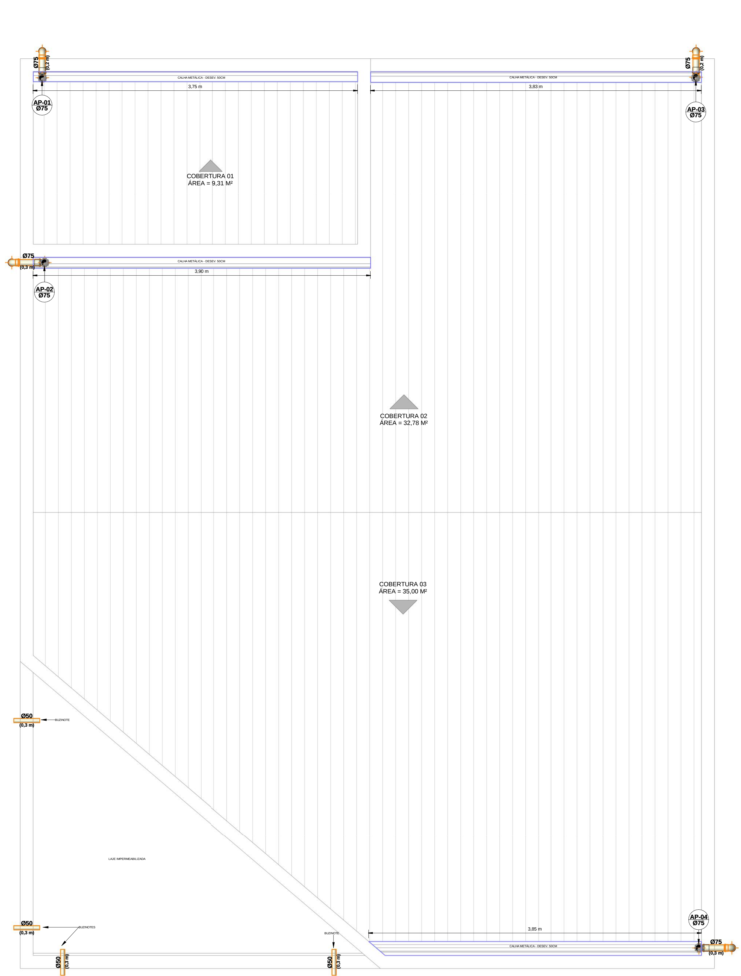
1 PLANTA DE COBERTURA - DRENAGEM PLUVIAL 1 : 25
