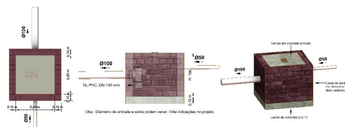
5 DET. CAIXA DE GORDURA 60X60cm 1 : 25
