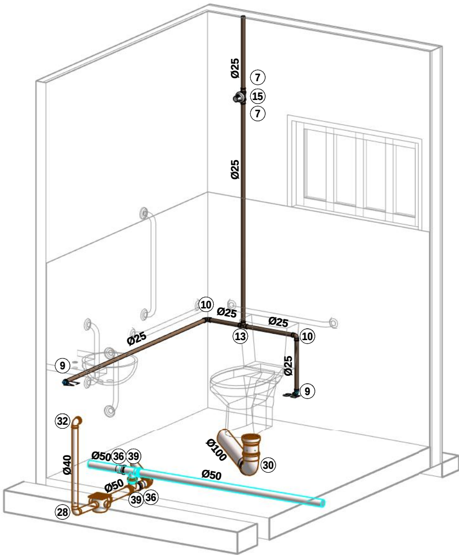
2 ISOMÉTRICA WC PNE FEM. 1 : 25
